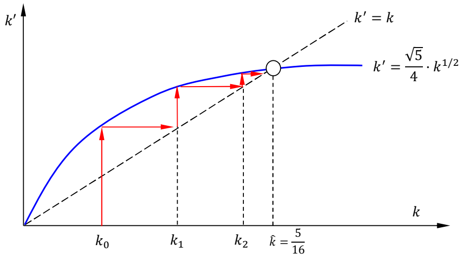
Fig. 1. Trajectòria del capital per càpita i estats estacionaris de la trajectòria ( k = 0 i k = \hat{k} = 5/16 )
